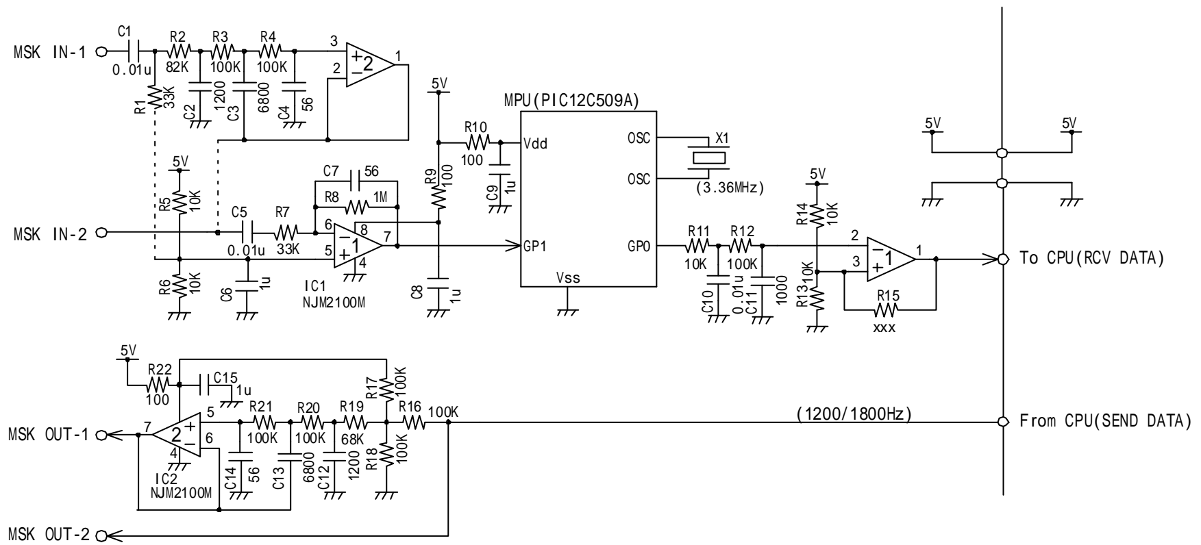
1200BPS MSK MODEM(案)
