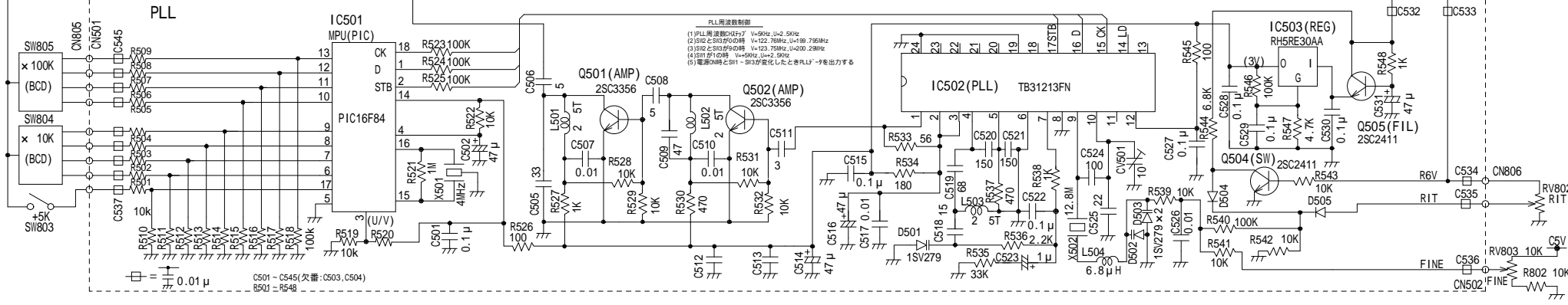
NTS210総合回路図(03版) 99.12.10
