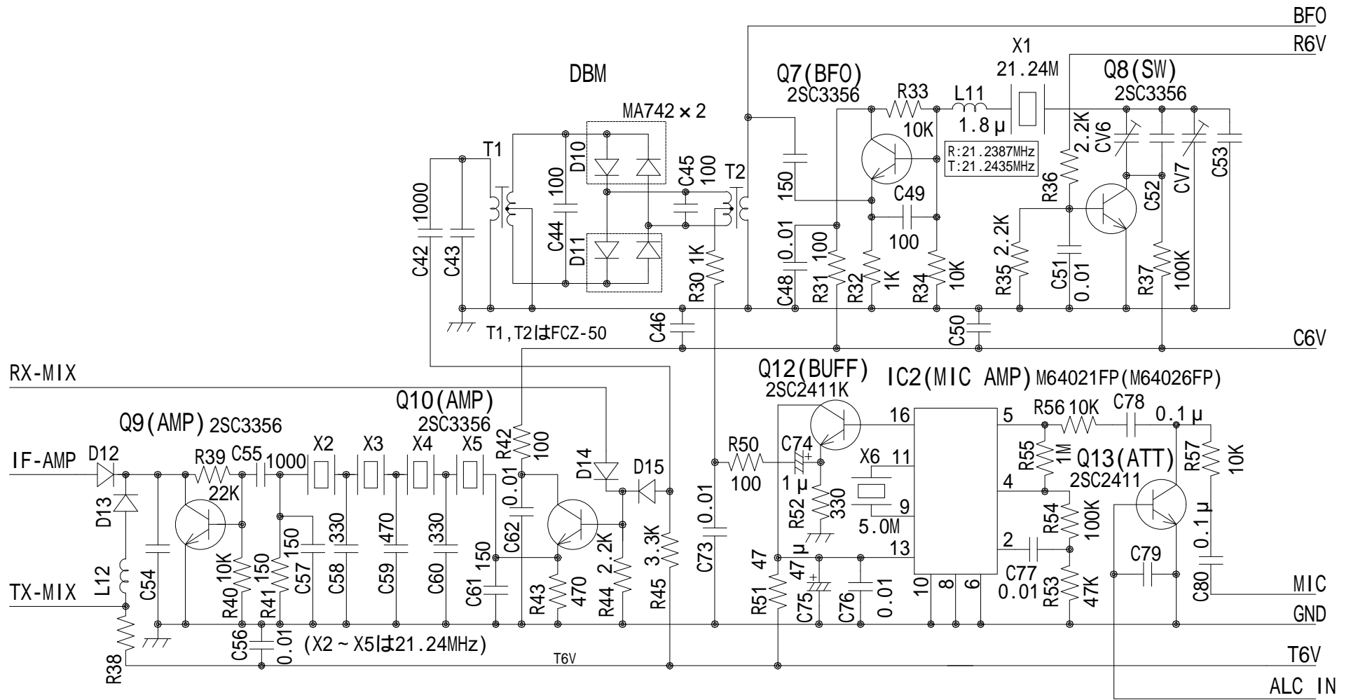
SSB GENERATOR 試作回路 (NTS210用)
