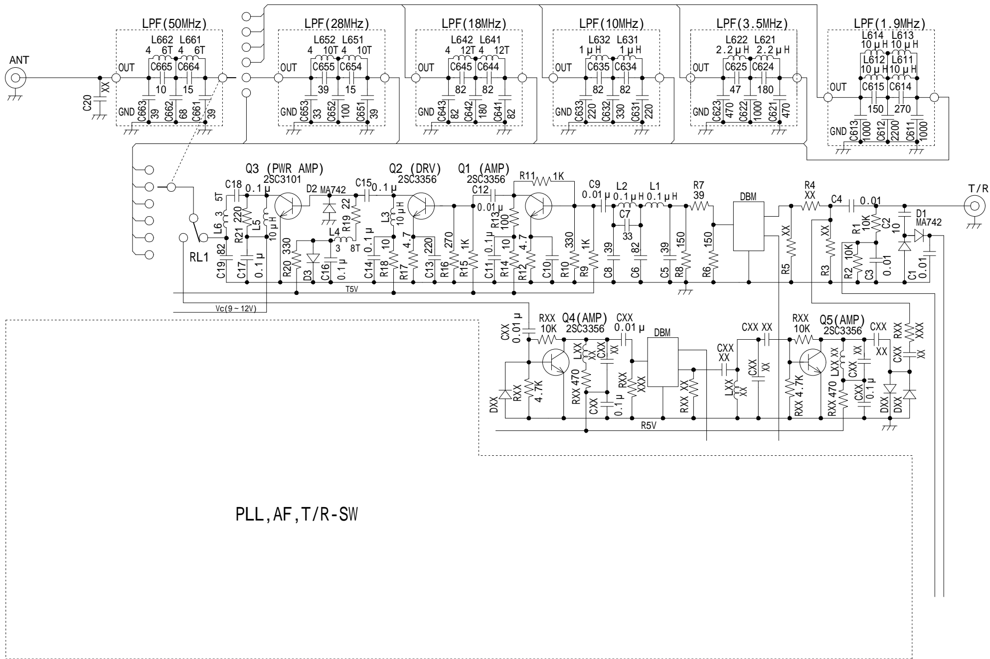
NTS-CO2A回路(1.8 ~ 54MHz, OUTPUT POWER=0.5 ~ 1W) (案)
