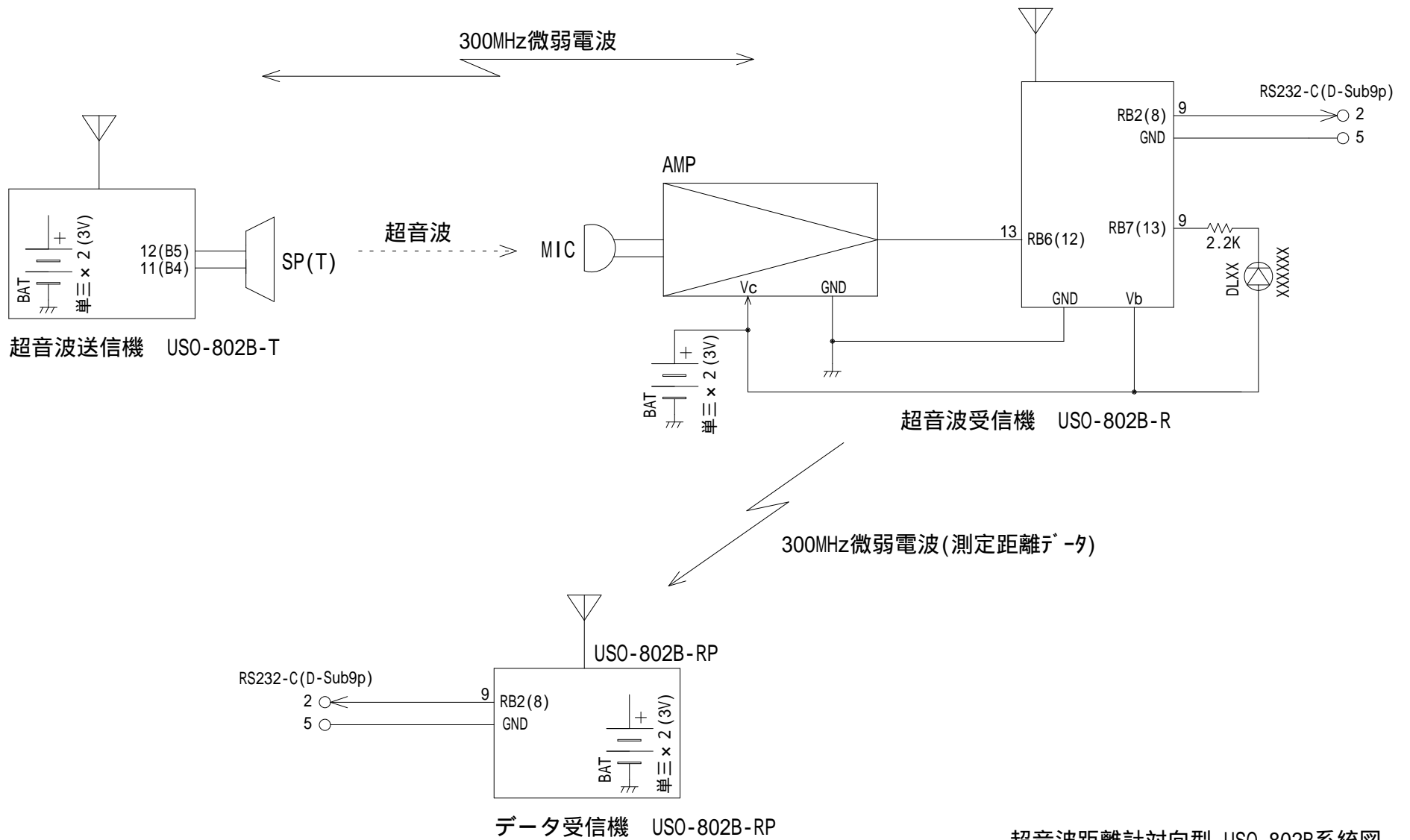
超音波距離計対向型-USO-802B系統図
